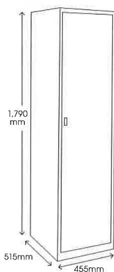
●外寸図
